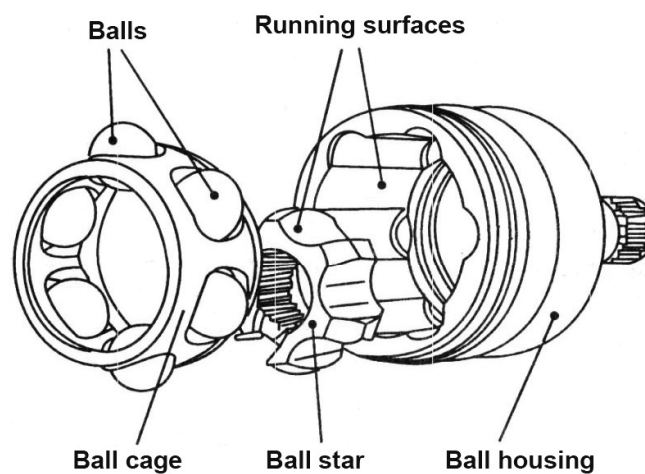
Fig. 4.1.9 Rzeppa Joint
